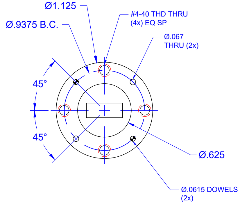
UG 425 FLANGE
