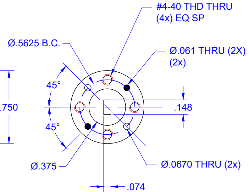
UG-385_FLANGE
